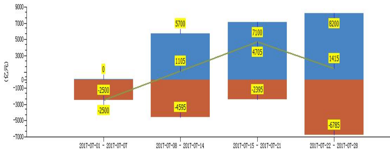
图 2: 股市走势
