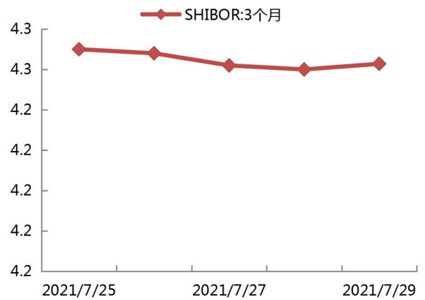
图 6: SHIBOR 走势
